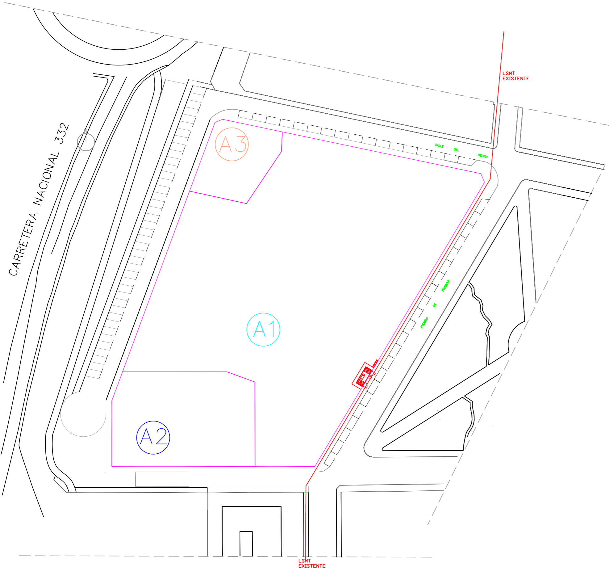
PLANO ACOMETIDA ELECTRICA
